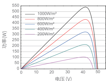
功率-电压曲线 JAM72D30-540/MB
